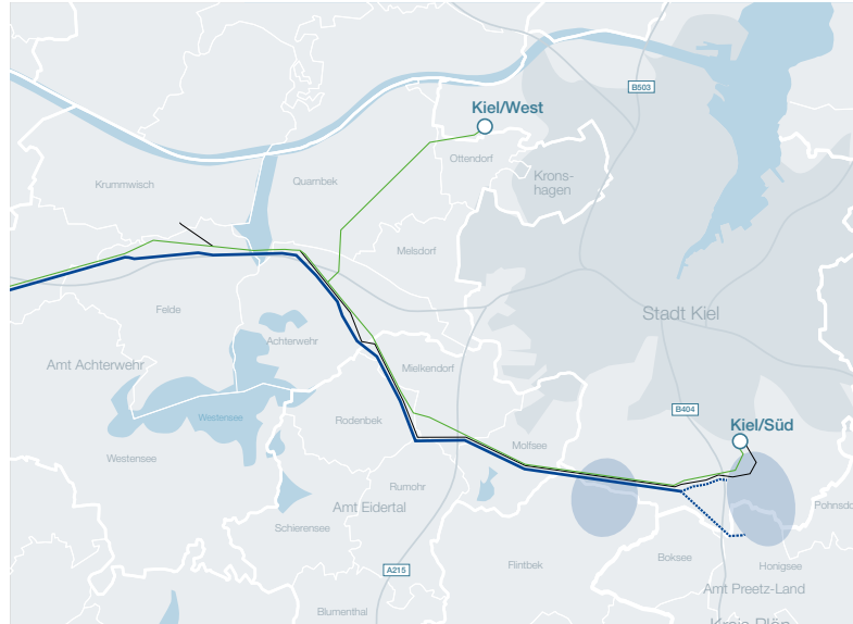
Die aktuelle Planung des Freileitungsbaus von Audorf bis zum Kieler Süden. Wo genau das neue, 30 Hektar große Umspannwerk entstehen soll, ist noch nicht geklärt. Die hellblauen Kreise markieren den Suchraum für das Umspannwerk.
